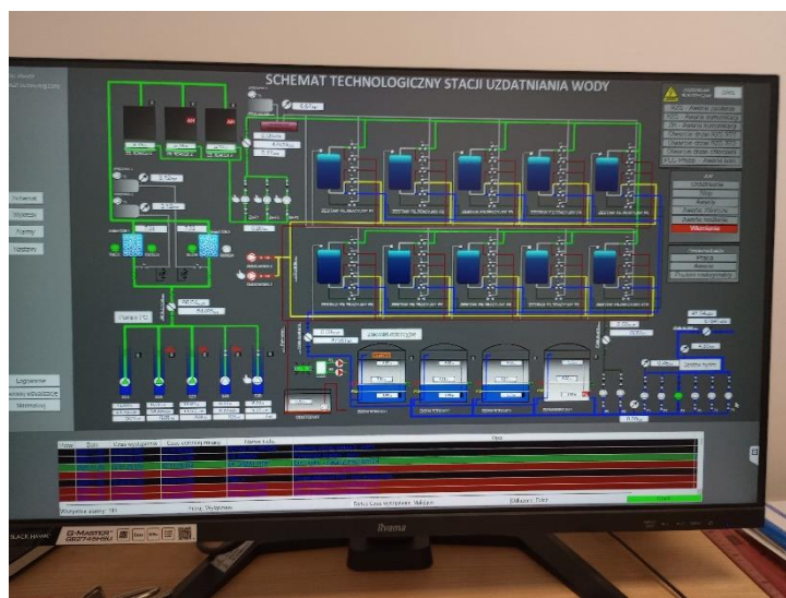
Schemat technologiczny stacji uzdatniania wody
